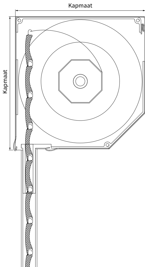
doorsnede kap
