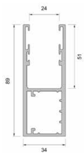
doorsnede UPH 89 geleider (G)
