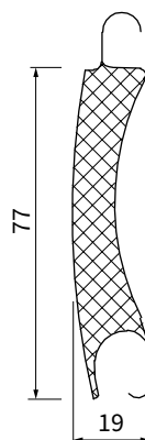
doorsnede lamel
