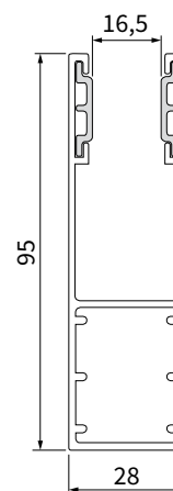
doorsnede UPH 260 geleider (G)
