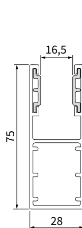
doorsnede UPH 240 geleider (G)
